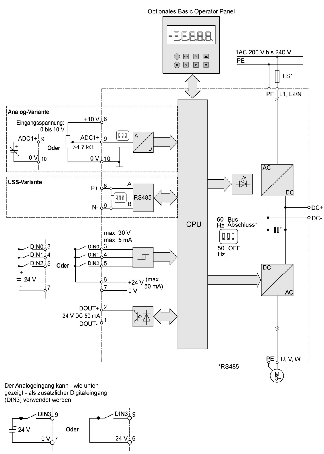
Рис. 2-2 Блок-схема
